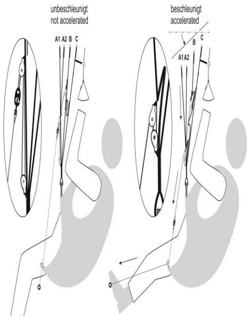
Fig. 12 Come lavora il sistema di velocità dell' ARCUS RS
