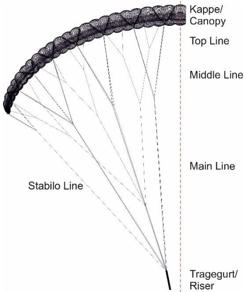
Fig. 1: CAD disegno ARCUS RS
