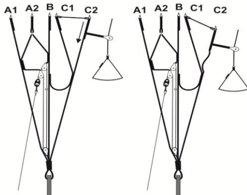
Fig. 6: Stabilizzatore a ponte sulle C
