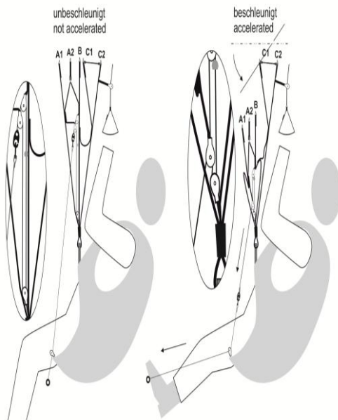
Fig. 12 Come lavora il sistema di velocità dell' AGERA RS
