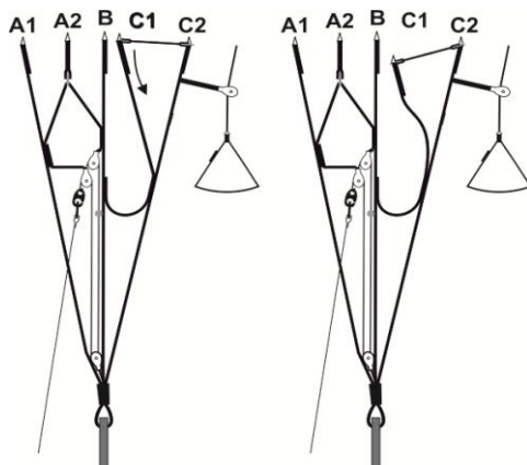
Fig. 7: Aggiustamento della direzione di volo tramite il ponte sulle C.
